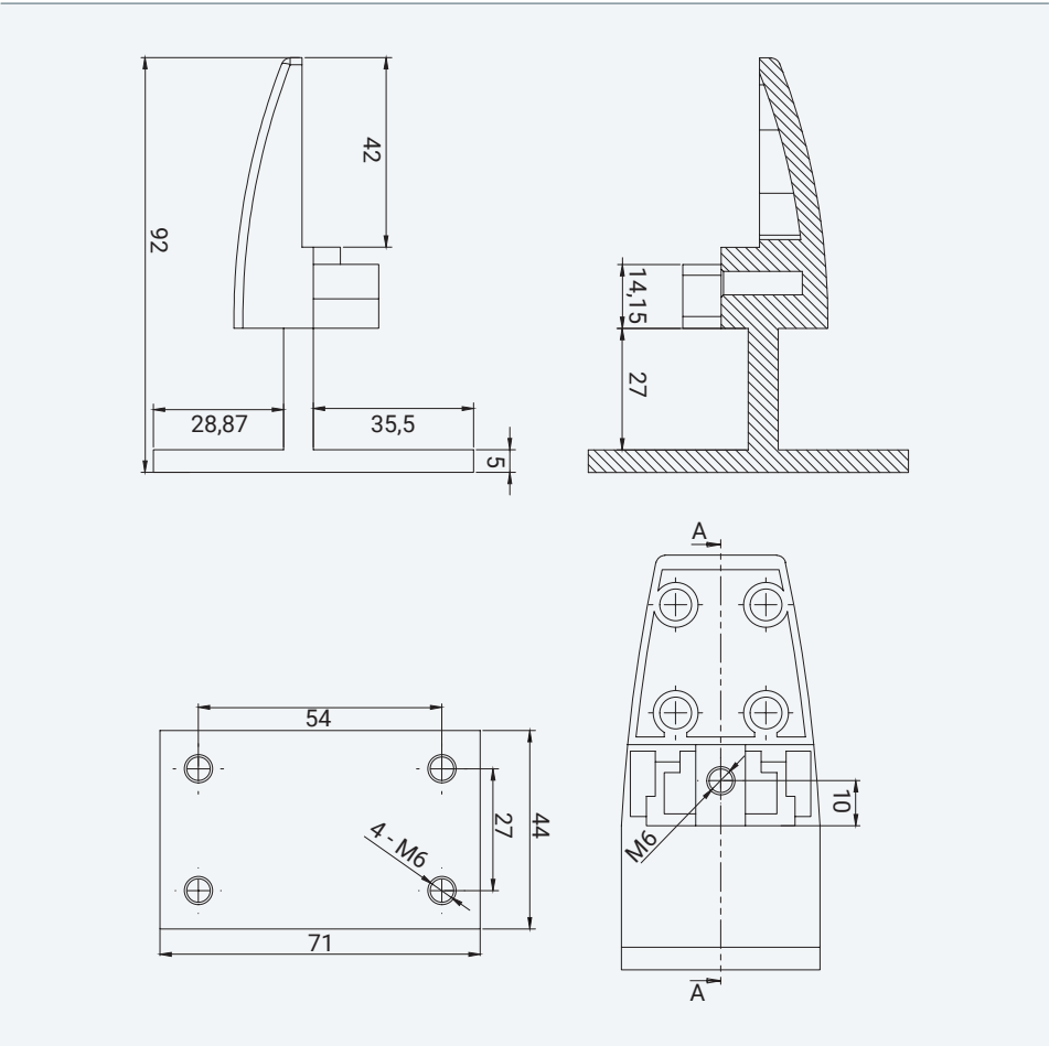
Technische Zeichnungen
