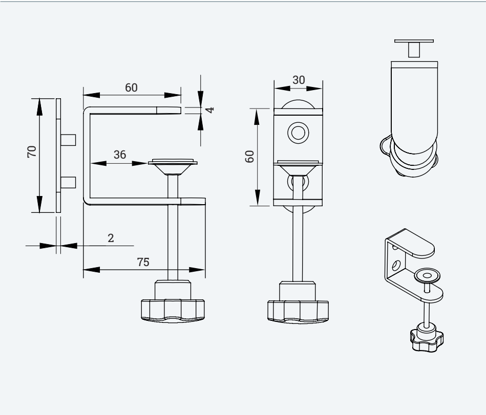
Technische Zeichnungen
