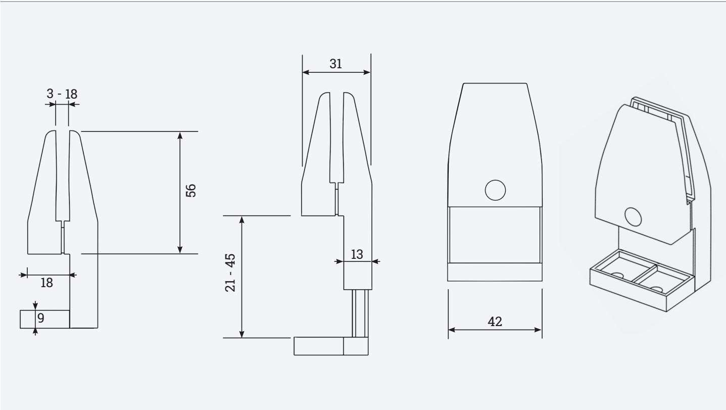
Technische Zeichnungen
