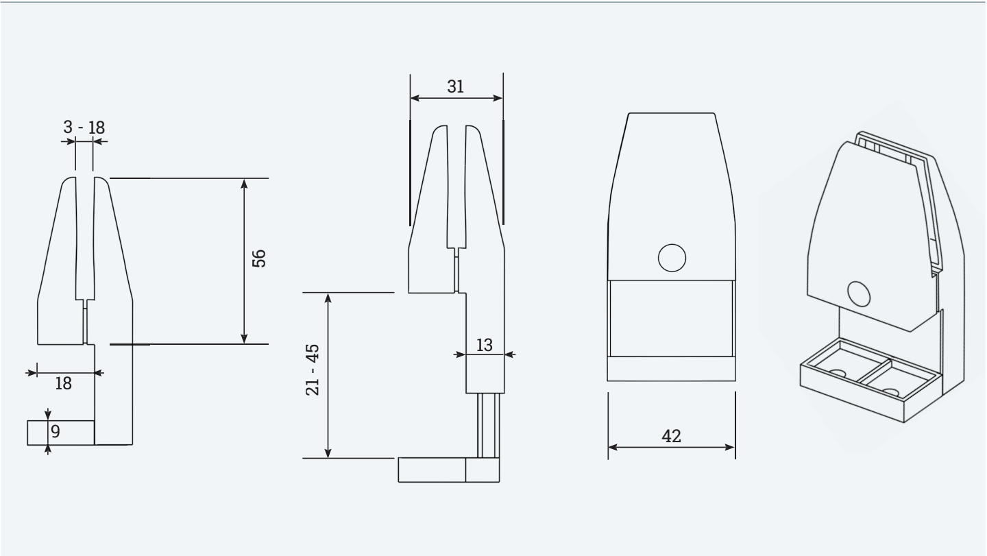
Technische Zeichnungen
