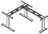
Montagevariante: A-90°
