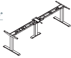
Montagevariante: B-Flex 60-180°
