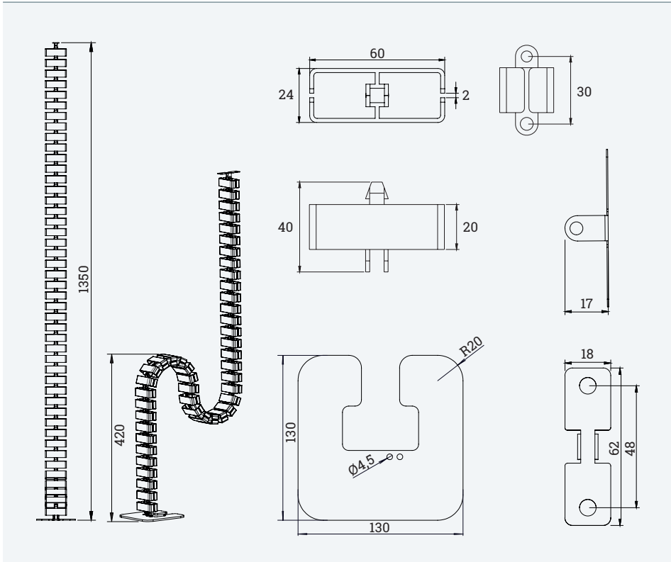
Einfaches Stecksystem
